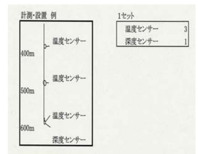
水深・水温調査の模式図
