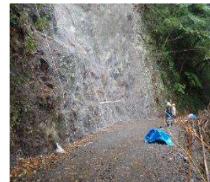
狭隘箇所のためロープ足場による施工を実施
